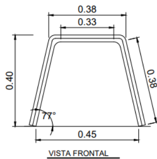
PIEZA # 5, ASIENTO Y PATAS TRASERAS
