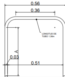
PIEZA METÁLICA 3 ESC. 1:10
