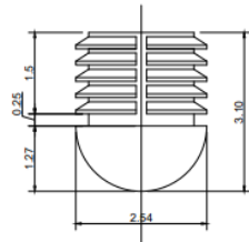
REGATÓN (SILLAS Y MESAS) O SIMILAR DE PLÁSTICO DE ALTA RESISTENCIA COTAS SE PRESENTAN EN CENTIMETROS
