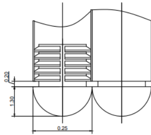
DETALLE DE PATAS DE DOS TUBOS CON REGATÓN
