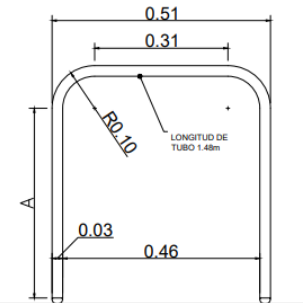
PIEZA METÁLICA 2 ESC. 1:10
