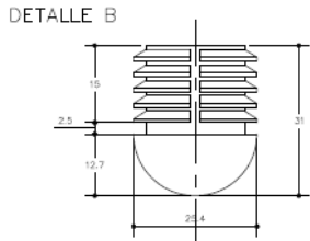
REGATON (SILLAS Y MESAS) O SIMILAR DE PLASTICO DE ALTA RESISTENCIA
