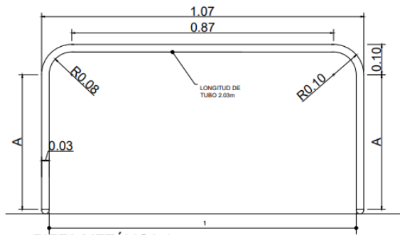
PIEZA METÁLICA 1 ESC. 1:10
