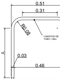
PIEZA METÁLICA 2 ESC. 1:10
