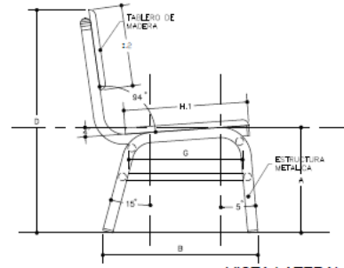
VISTA LATERAL
