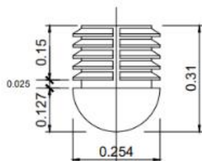
REGATON O BOTA DE HULE (sillas y mesas)
