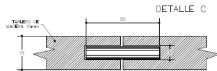
UNION ENTRE TABLEROS CON TACOS DE MADERA
