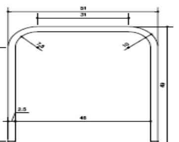
PIEZA METÁLICA 2
