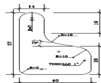
PIEZA # 3 BRAZO DE MADERA
