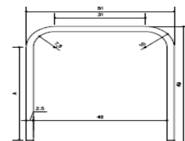
PIEZA METÁLICA 2
