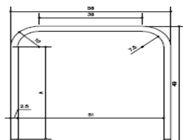
PIEZA METÁLICA 3
