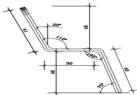
VISTA LATERAL. PATAS DELANTERAS.
