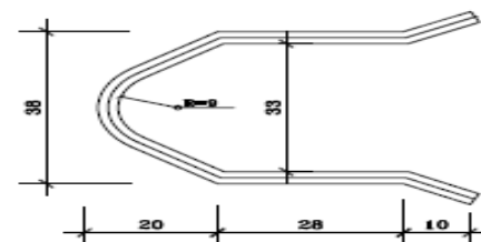
VISTA SUPERIOR. ASIENTO.
