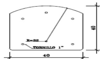
PIEZA # 2 ASIENTO DE MADERA
