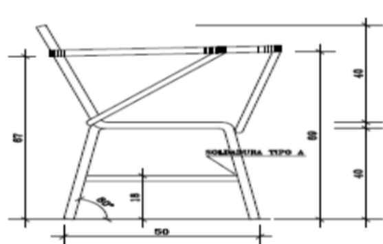
VISTA LATERAL
