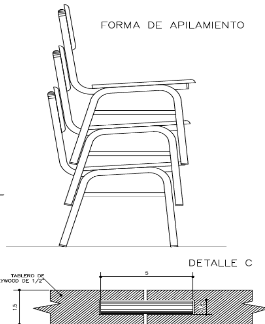
UNIÓN ENTRE TABLEROS CON TACOS DE MADERA
