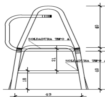
VISTA FRONTAL ESCALA 1:10
