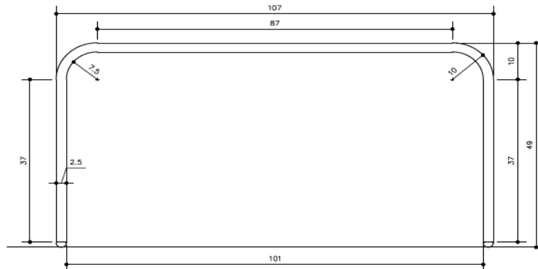
PIEZA METÁLICA 1
