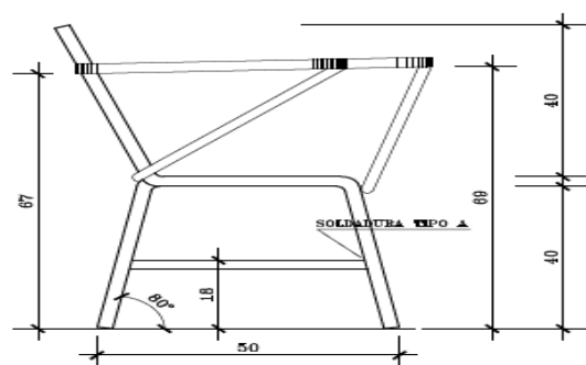
VISTA LATERAL ESCALA 1:10
