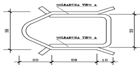
VISTA SUPERIOR ESCALA 1:10
