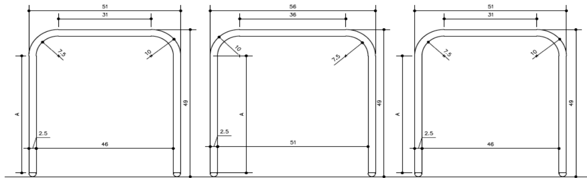
PIEZA METÁLICA 2
