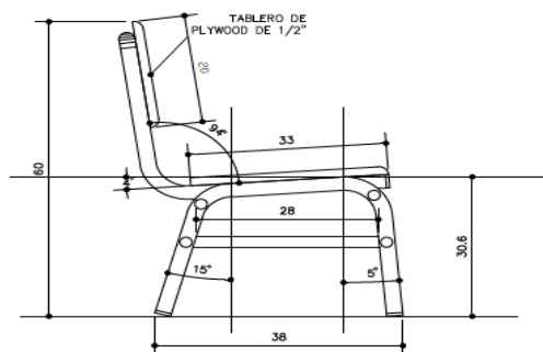
VISTA LATERAL
